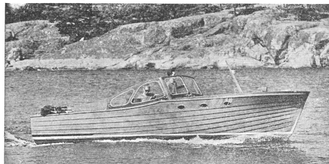
SOLÖ 7,25 x 2,25 m, den populära ruffbåten med 3 kojplatser, garderob och pentry. Motor: Volvo Penta BB 70, fart ca 17 knop, eller MB 18 F, fotogen med direktstart, fart ca 16 knop.
