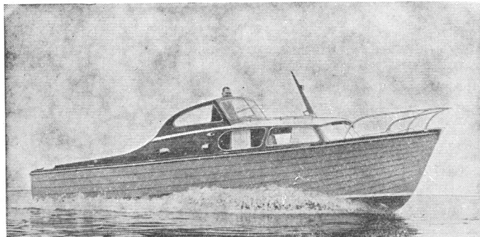
BERGÖ cabinkryssare 7,80 x 2,54 m, 4 kojplatser, toalett och pentry. Motor: Volvo Penta BB 100, ca 16 knop, MB 18 F, fotogen med direktstart, ca 13 knop.
