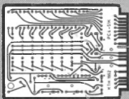
TRYCKT LEDNINGSDRAGNING
